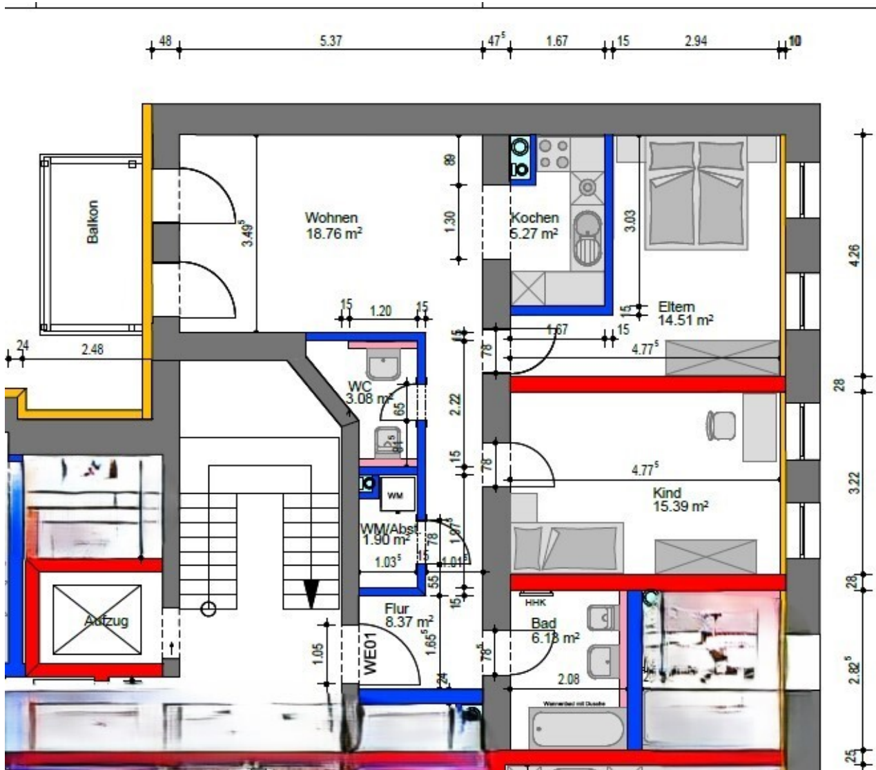
Grundriss WE 01
